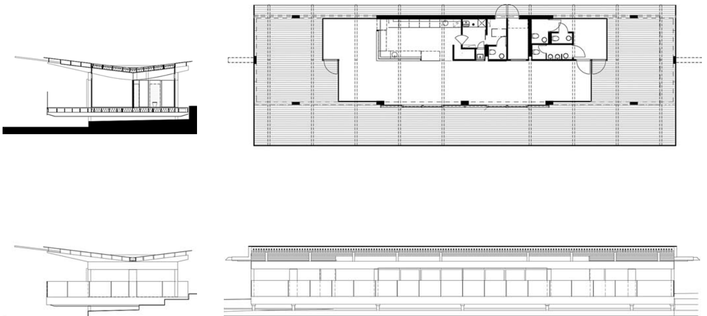
Julkisivut, pohjapiirustus ja leikkaus1:300
