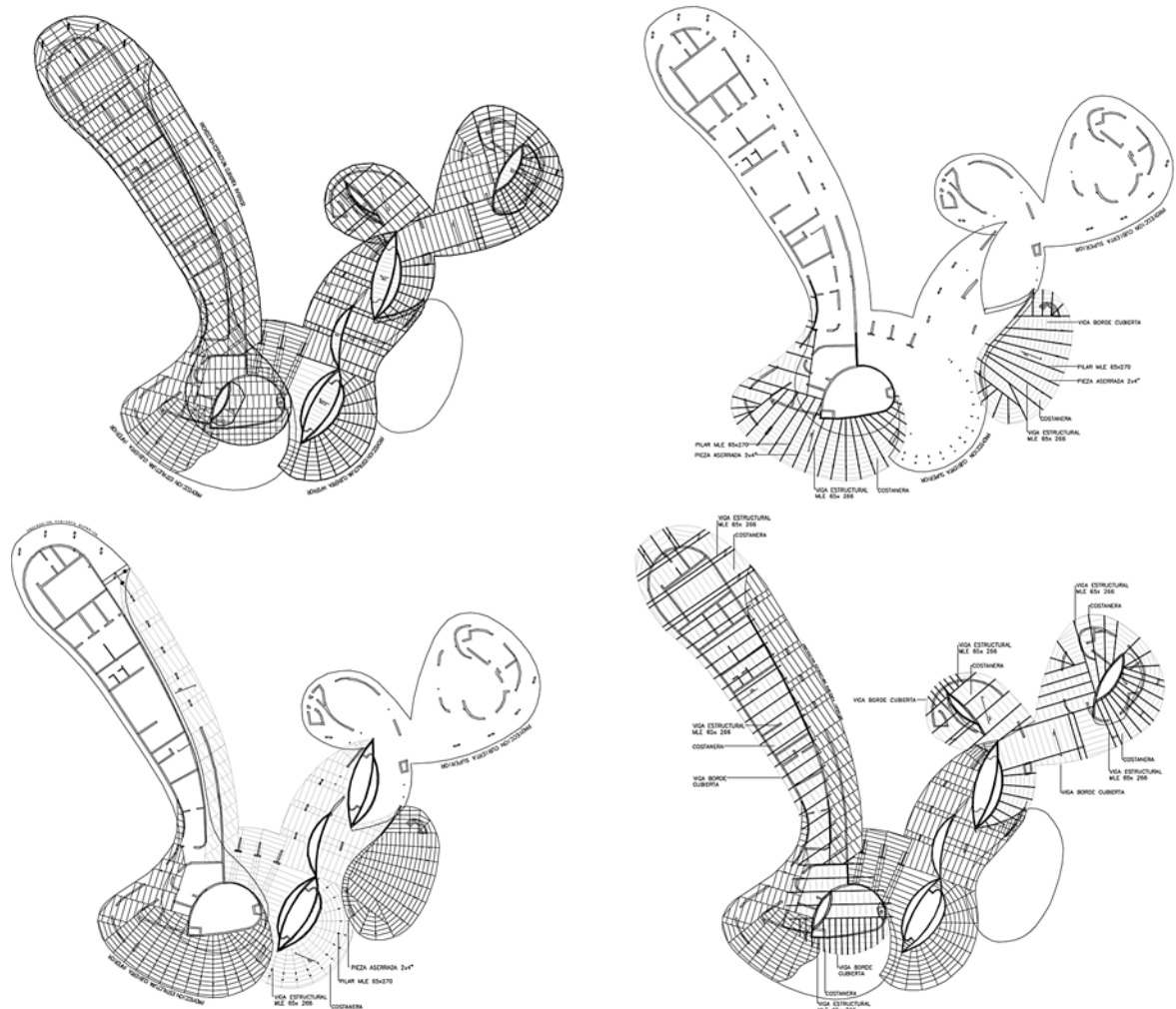
Pohjapiirustukset 1:1000 Hotelli Explora, Pääsiäissaaret, 2008
