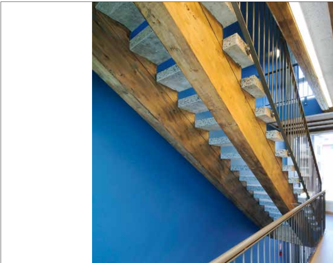
Kuva 54. Portaan B-s1, d0-luokan puurakenteiset kannatinpalkit eivät tarvitse suojaverhousa P2-paloluokan puukerrostalossa (vähäinen rakennusosa). Kuva: Metsä Wood.
