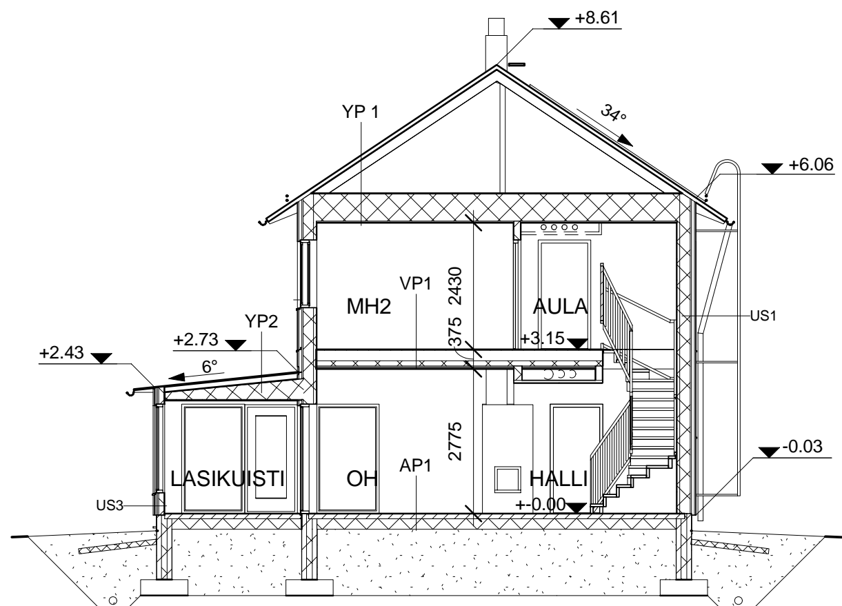
LEIKKAUS A-A 1 : 100
