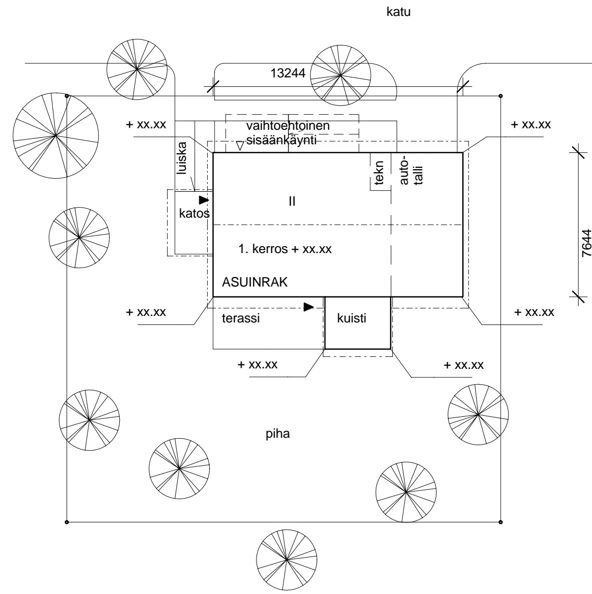
TONTTIKAAVIOT TALOMALLI 3A SIJOITETTUNA n. 400m 2 TONTILLE MITAT SUUNTAAN ANTAVIA
