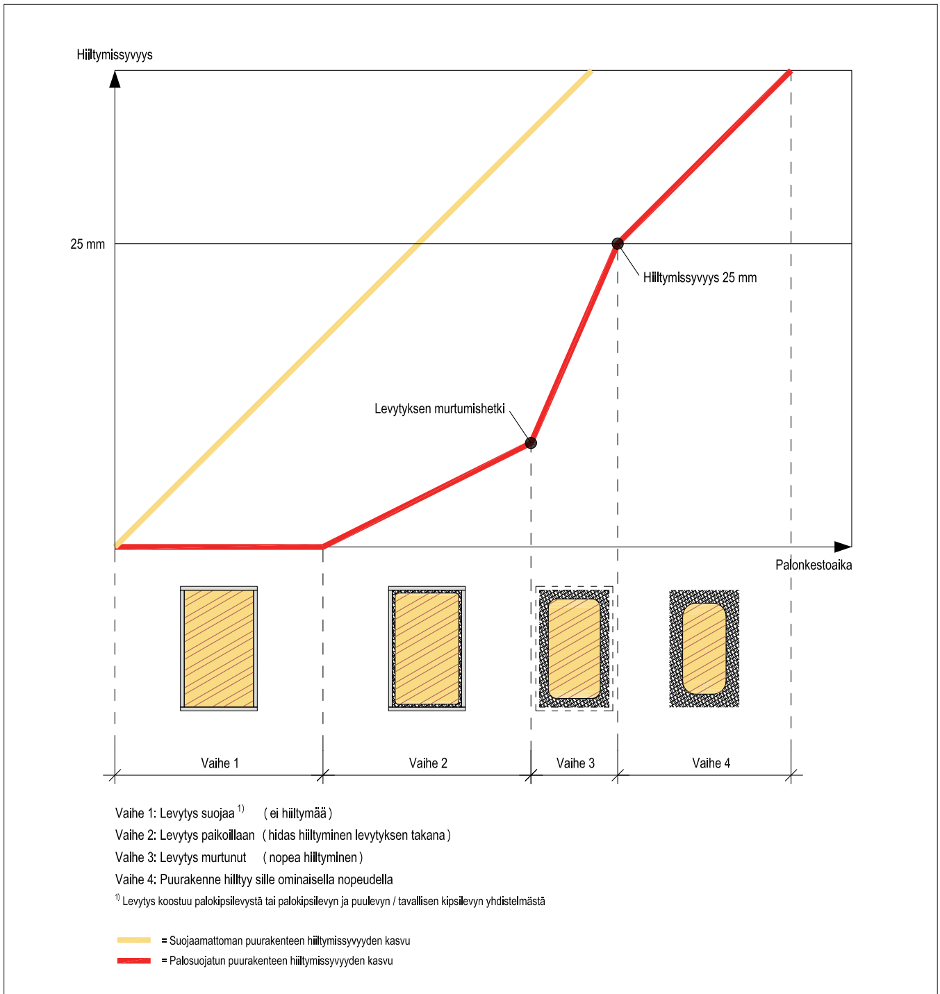
Kuva 77. Hiiltemisyvyyskasvu ajan funktiona, kun puurakenteen hiiltymisen alku on ennen palosuojauksen murtumista ja hiiltymisnopeus palautuu suojaamattoman puun hiiltymisnopeuteen puurakenteen saavutettua 25 mm:n hiiltemisyvyys.
