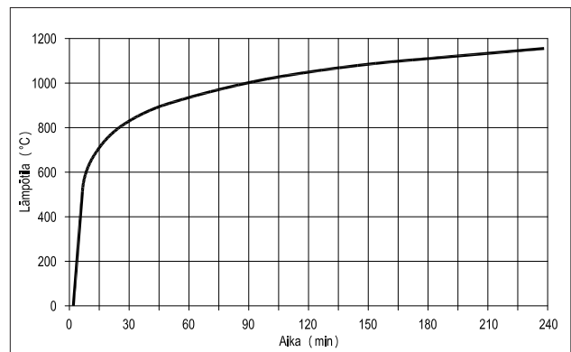
Kuva 5. Standardipalokäyrä.
