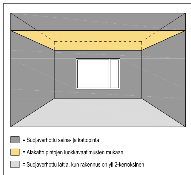
Kuva 18. Suojaverhoitus tilaa rajoittavissa pinnoissa.
