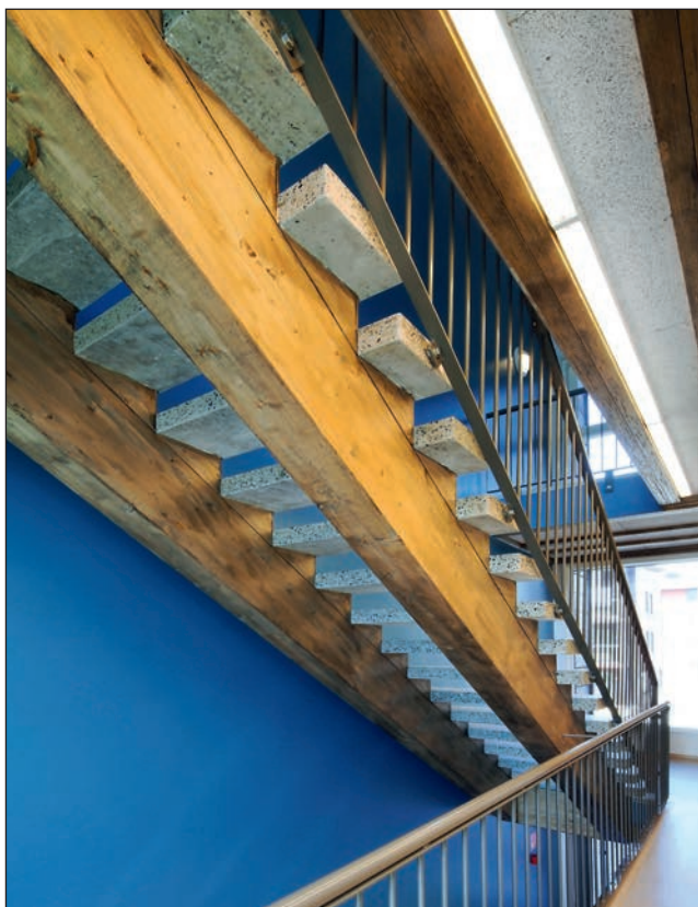
Kuva 60. Portaani B-s1, d0-luokan puurakenteiset kannatinpalkit eivät tarvitse suojaverhusta P2-paloluokan puukerrostalossa (vähäinen rakennusosa). Kuva: Metsä Wood
