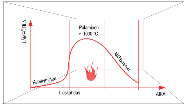
Kuva 2. Palon kehittymisen yleiskuvaus sprinklaamattomassa asuinhuoneistossa.
